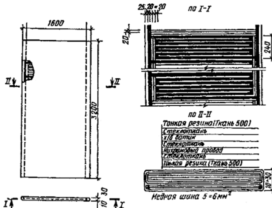
Рис.2. Термoeлектрический мат
