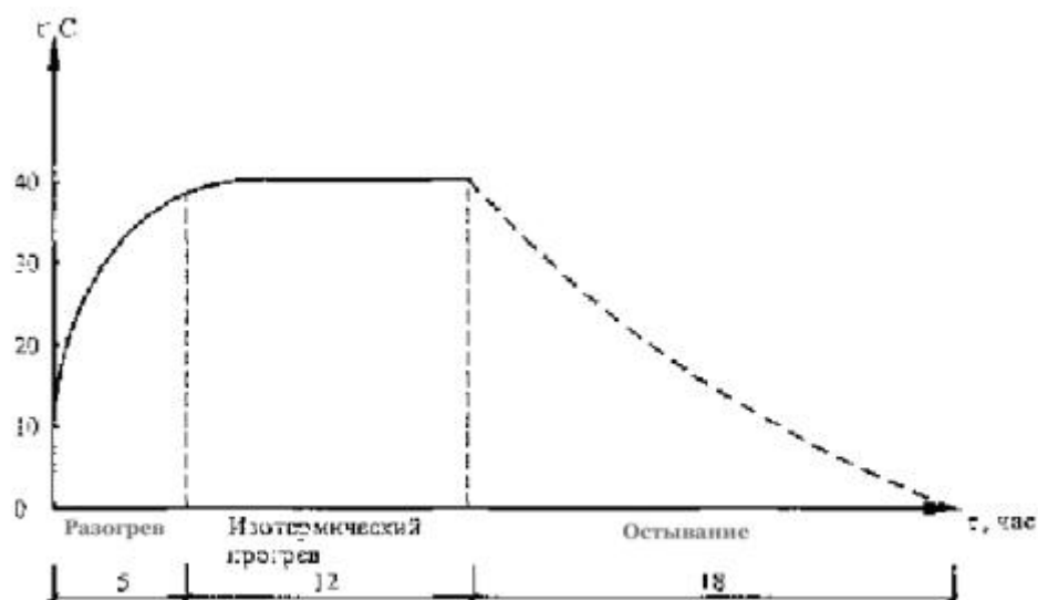
Рисунок 7 - График температурного режима электродного прогрева конструкции
