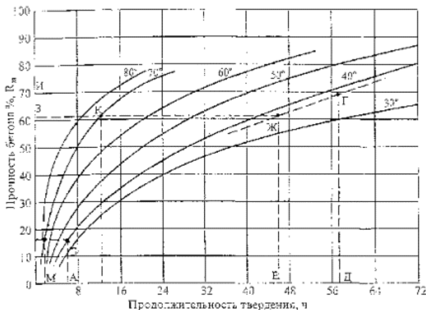
Рисунок 9 - Пример определения прочности бетона по графику
