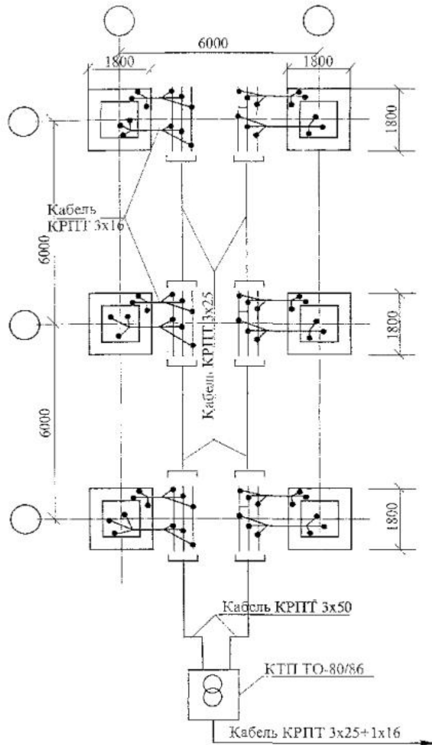
Рисунок 4 - Схема подключения шинпроводов к питающей сети
