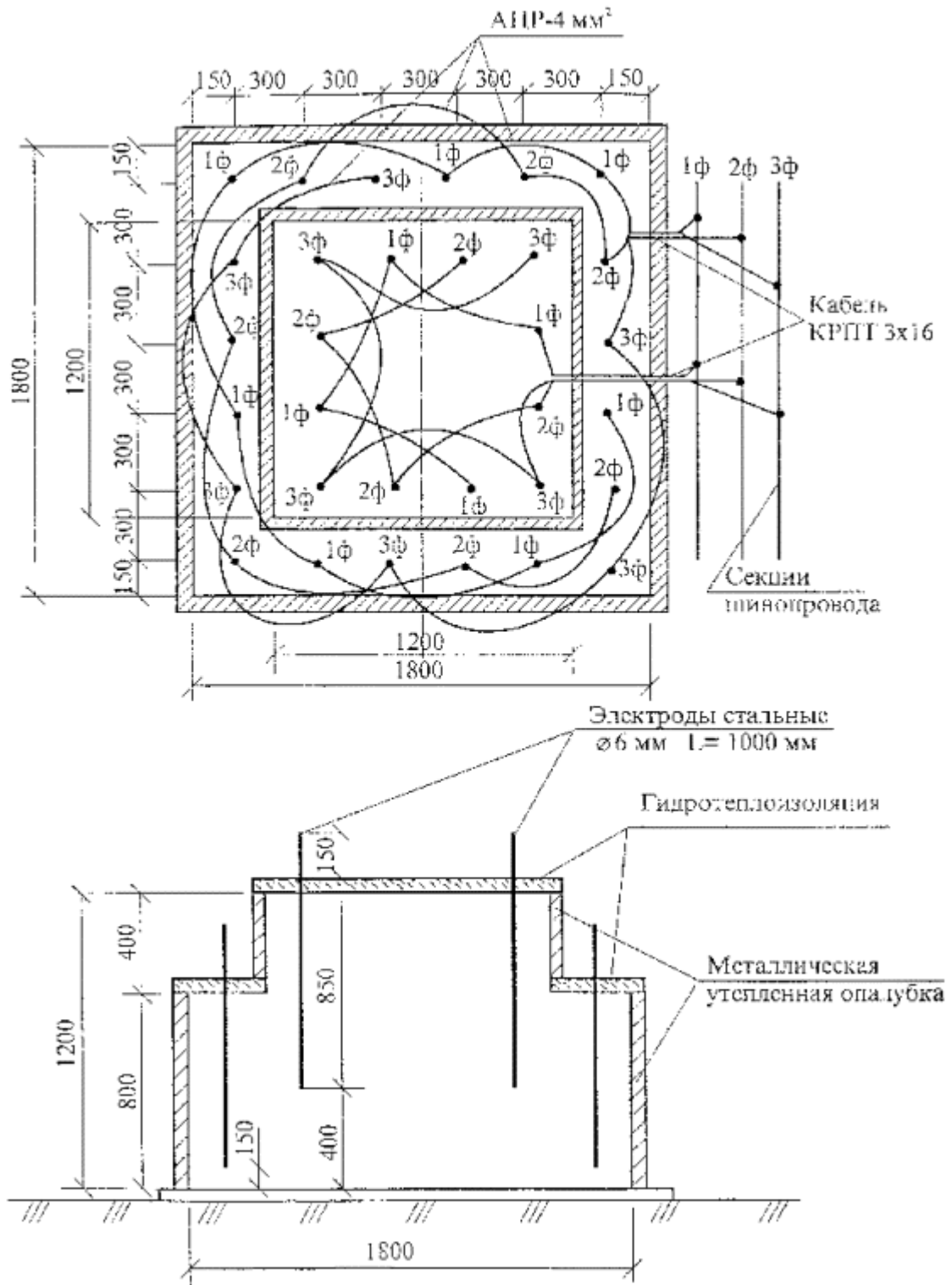
Рисунок 3 - Схема установки электродов и подключения к шинопроводам
